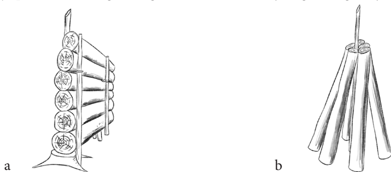
Ryc. 2. Stos kontrolny w kształcie ściany (a) i stożka (b)
